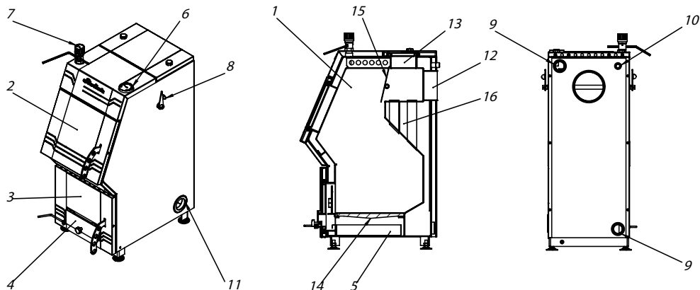
Рисунок - 2. Устройство аппарата отопительного.
