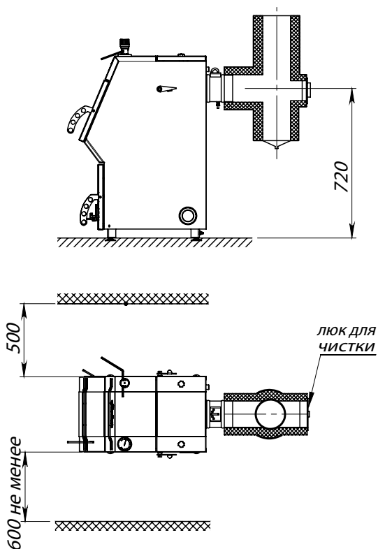
Рисунок - 3. Схема установки аппарата
