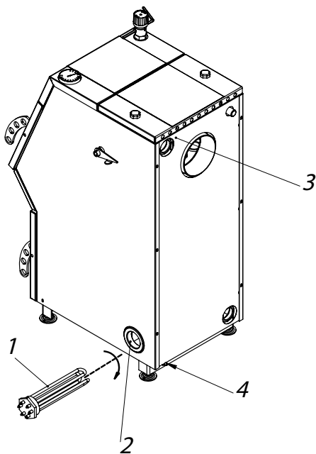
Рисунок - 4.2 Установка блока ТЭН на аппарате
