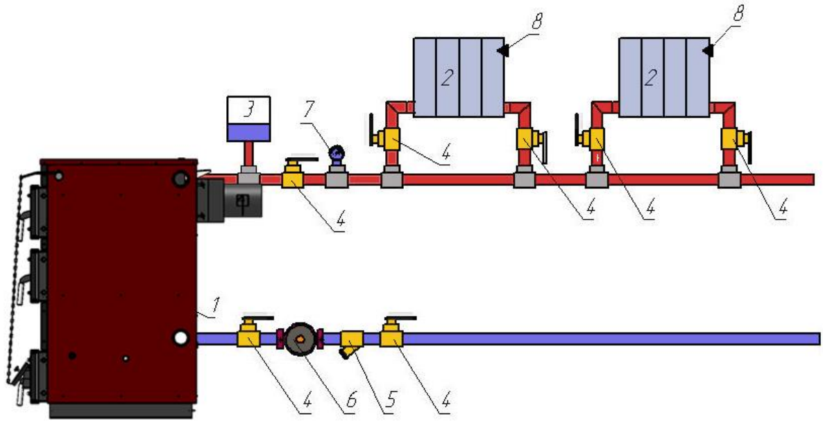
Рис. 5 Схема подключения котла к однотрубной открытой системе с принудительной циркуляцией теплоносителя 1 – котел, 2 – радиатор отопления, 3- расширительный бак, 4 – кран шаровый, 5 – сетчатый фильтр, 6 – циркуляционный насос, 7 – прибор учета давления, 8 – кран для спуска воздуха.
