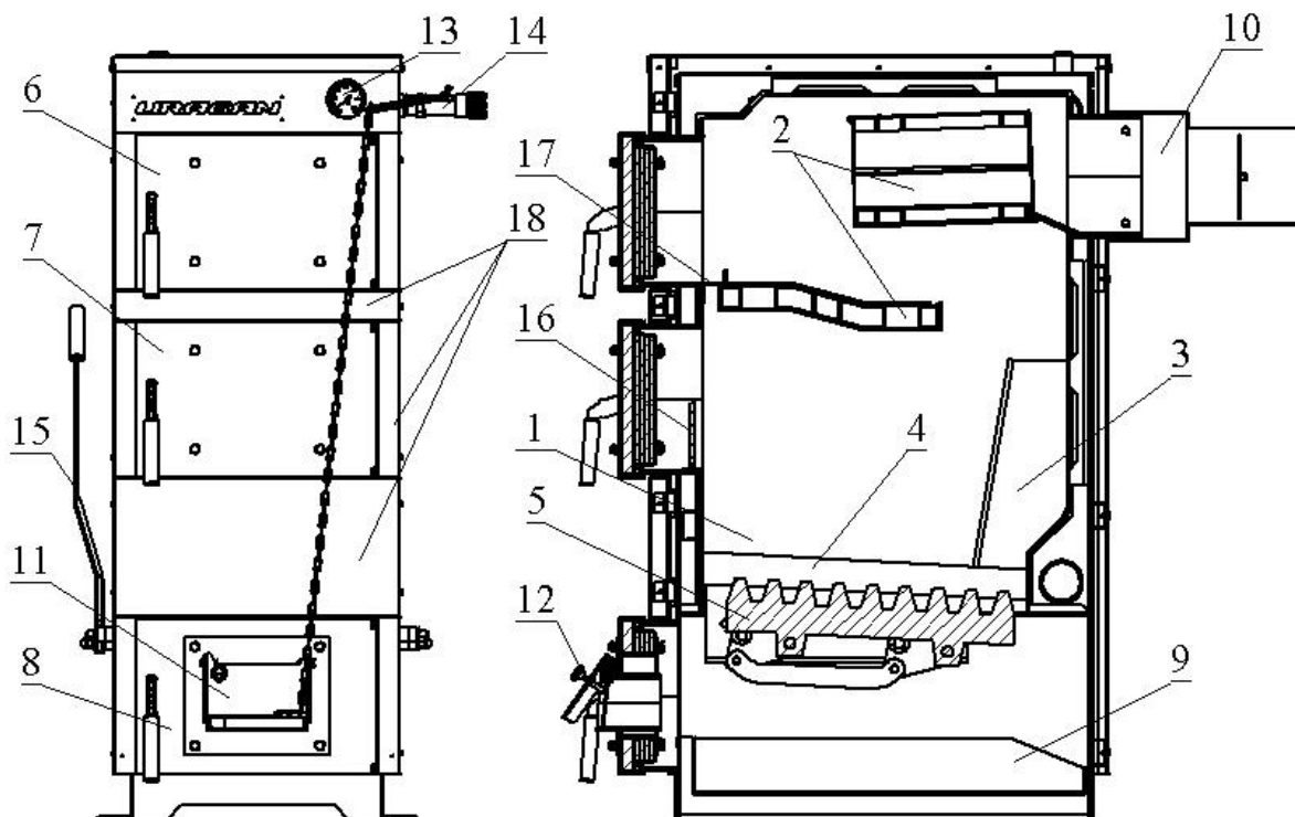
Рис. 1 Устройство котла
