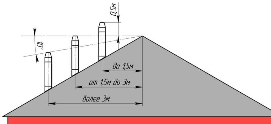
Рис. 2 Высота дымохода.
