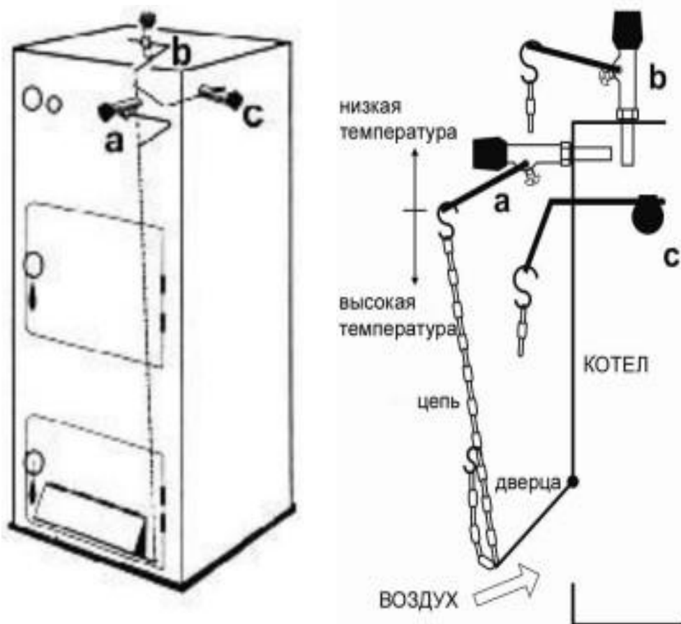
Рис. 7 Установка и калибровка регулятора тяги
