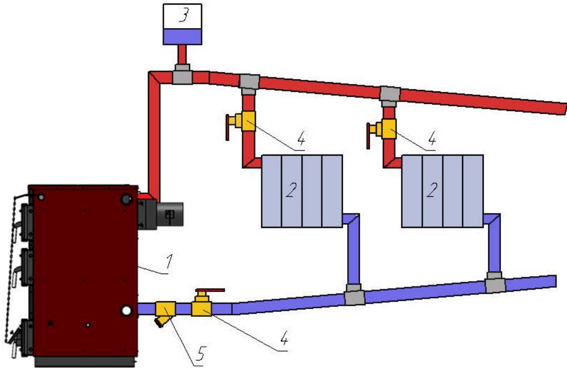
Рис. 3 Схема подключения котла к открытой системе с естественной циркуляцией теплоносителя.
