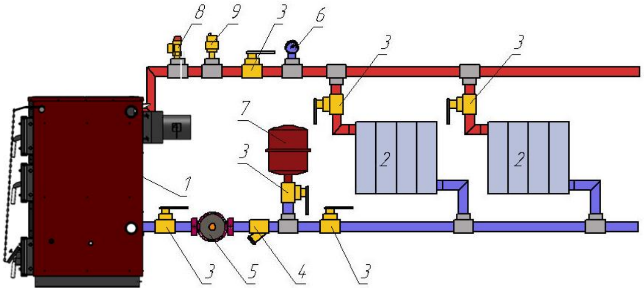
Рис. 6 Схема подключения котла к двухтрубной закрытой системе с принудительной циркуляцией теплоносителя 1 – котел, 2 – радиатор отопления, 3- кран шаровый, 4 – сетчатый фильтр, 5 – циркуляционный насос, 6 – прибор учета давления, 7 – расширительный бак мембранного типа, 8 – предохранительный клапан 1,5бар, 9 – автоматический воздушный клапан.
